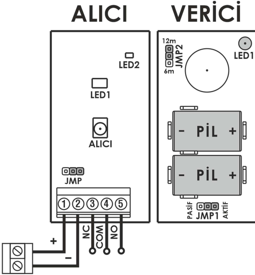
Şekil 7.1 EMFP Bağlantı Şeması
