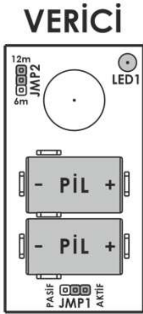
Şekil 4.1 EMFP-V Kontrol Kartı
