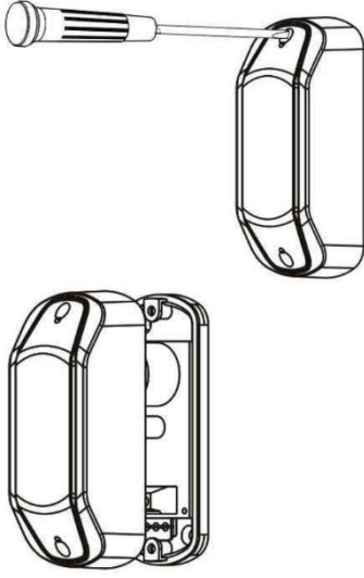
Şekil 6.1 – Adım 1: EMFP ön kapağın sökülmesi.
