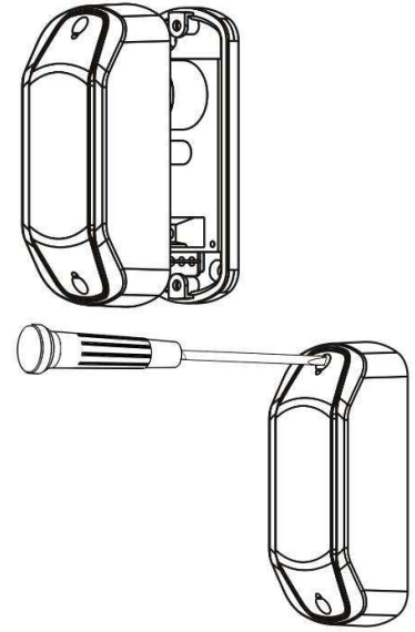
Şekil 6.5 – Adım 5: EMFP ön kapağının takılması.
