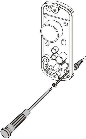
Şekil 6.3 – Adım 3: EMFP duvara montajı.
